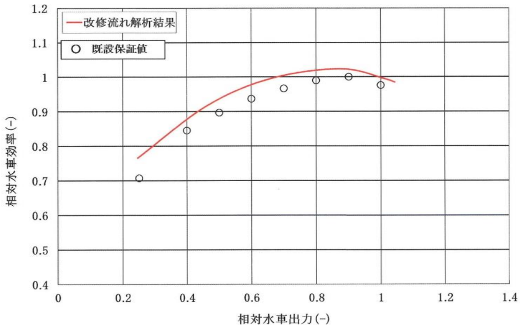
図1.水車効率比較
