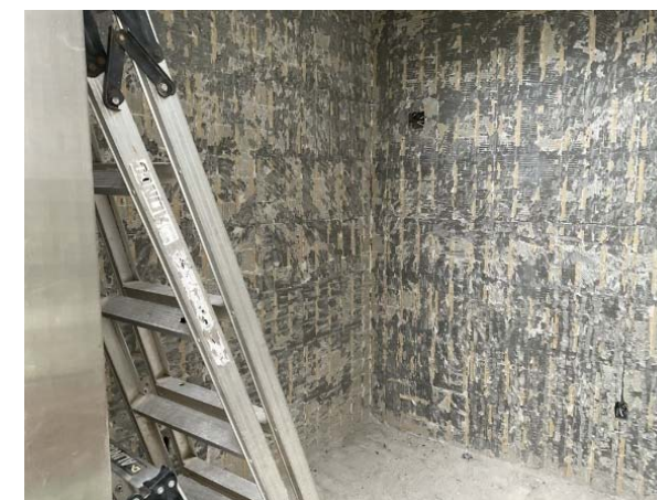
屋外トイレ内の器具類及び内壁の撤去状況
