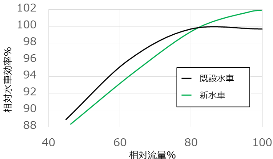
図1 水車効率向上効果
