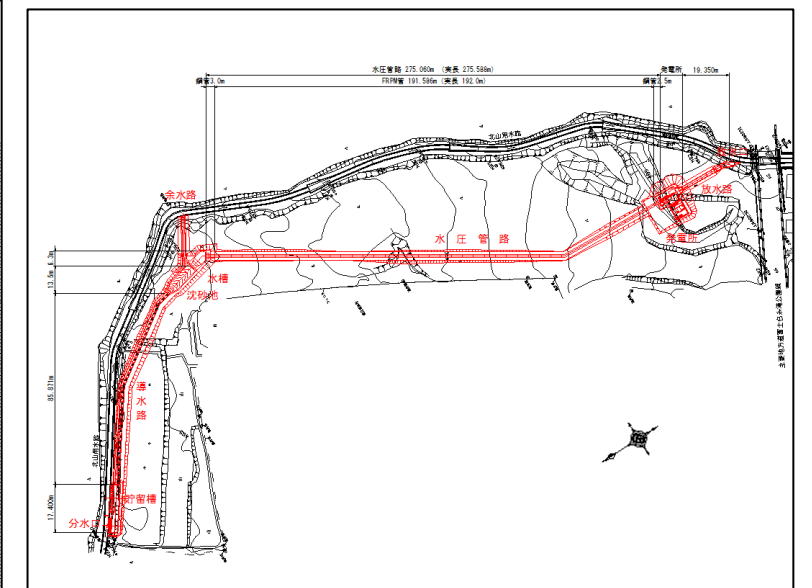
基本設計平面図
