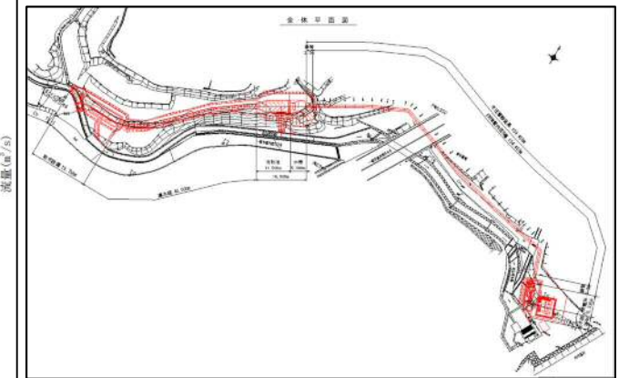
基本設計平面図
