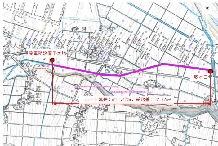
取水ルート図
