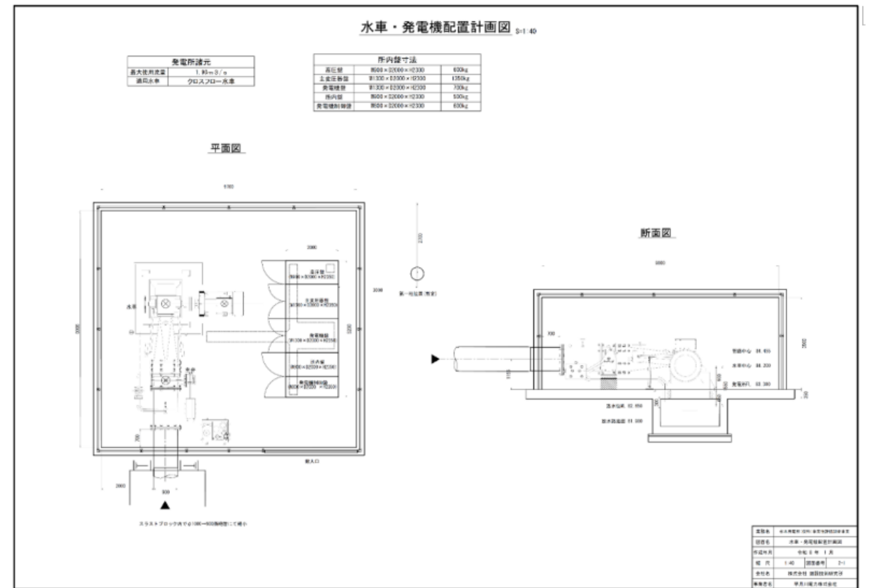
水車・発電機計画図
