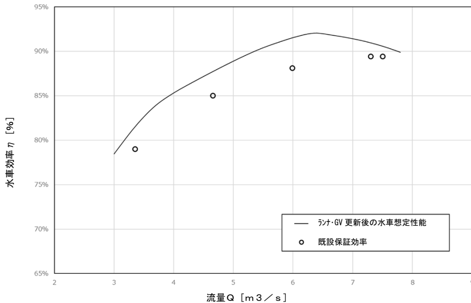
図. 水車効率比較（最高有効落差時）
